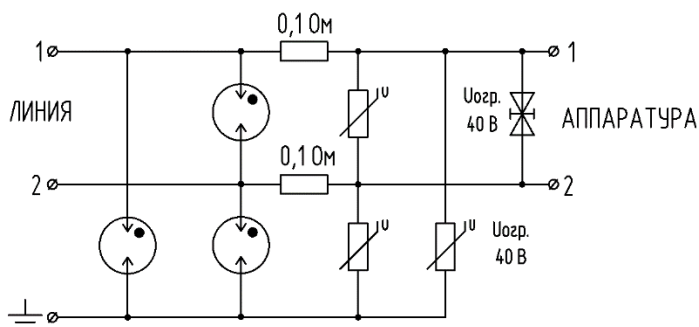
Рисунок 3.1 - УЗИП БГр-24-VAC Рисунок 3.2 Схема электрическая УЗИП БГр-24-VAC
